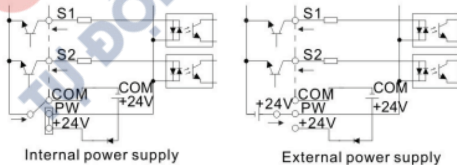
Hình 3-12 Kiểu NPN
