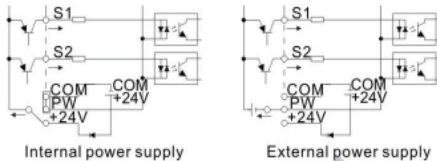
Hình 3-13 Kiểu PNP
