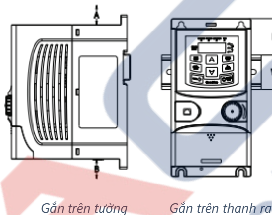
Hình 3-1 Lắp đặt
