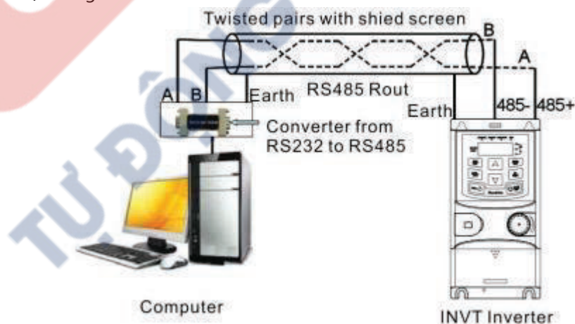
Hình 1: Kết nối vật lý RS485 trong truyền đơn
