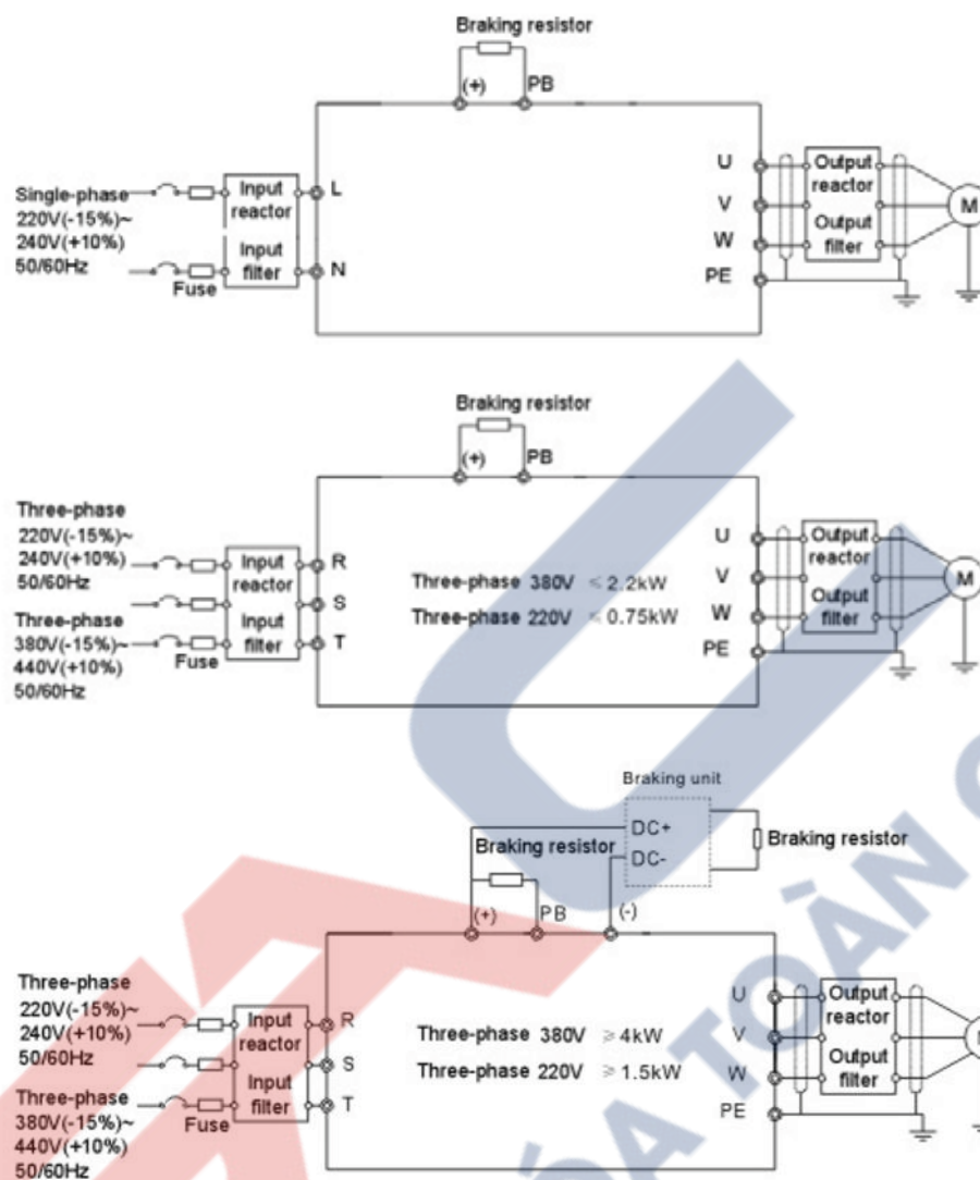
Hình 3-3 Sơ đồ đấu dây mạch chính
