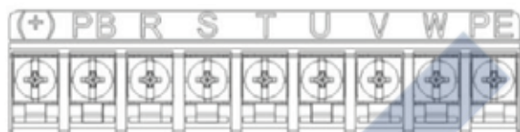
Hình 3-5: 3PH Terminal mạch chính (220V, \leq 0.75kW , và 380V, \leq 2.2kW )
